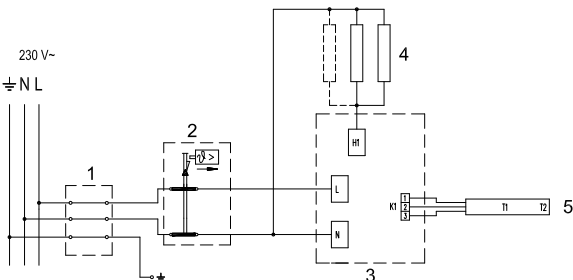
Рис. 5: Електросхема
